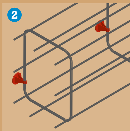
Standaard Wapeningskorf
