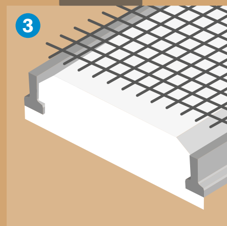
Combinatievloer
