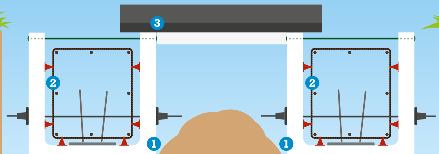
Standaard Wapeningskorf
